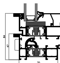
okno otvíravé – řez
