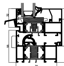
okno otvíravé – řez MB-70 HI
