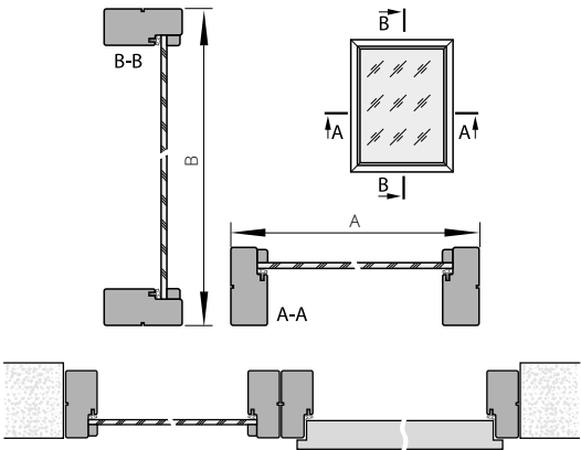
FALCOVÝ SYSTÉM
