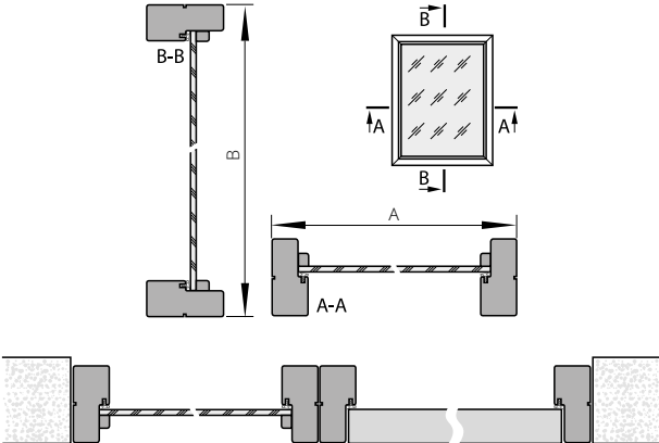
BEZFALCOVÝ SYSTÉM
