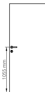
VÝŠKA KLIKY
