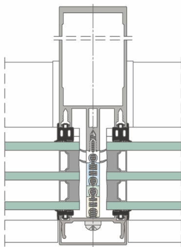
ŘEZ SLOUPKEM FA 50N
