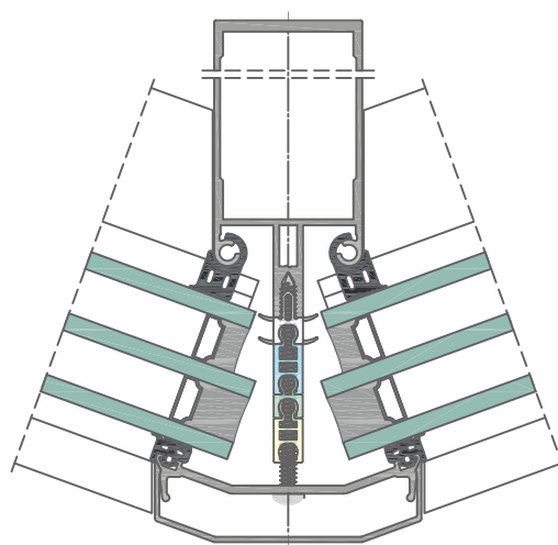
PŘÍČNÝ ŘEZ ÚHLOVÉ KONSTRUKCE FA 50N
